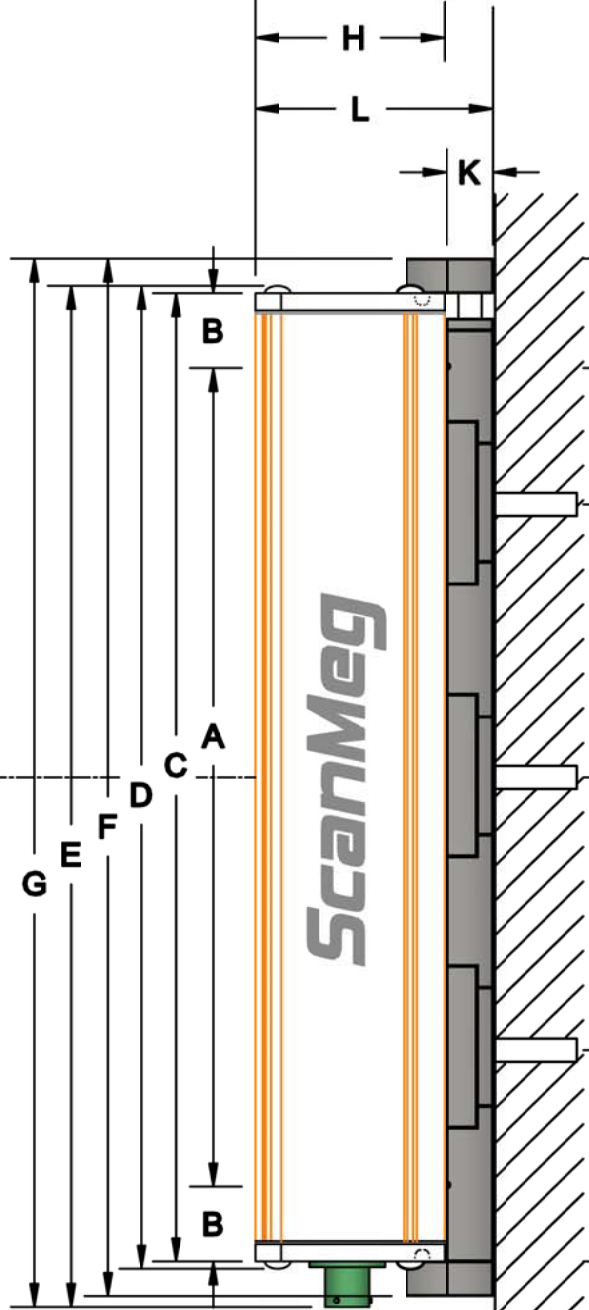
Side View with Bracket Vue de coté avec support
